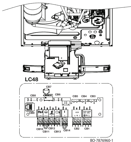
Εικ.46 Σύνδεσεις πλακέτας λέβητα
