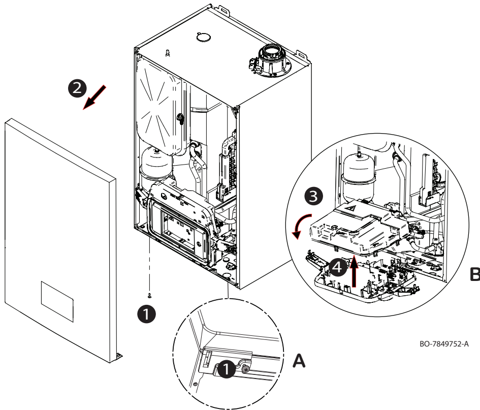
Εικ.45 Πρόσβαση στις ηλεκτρικές συνδέσεις
