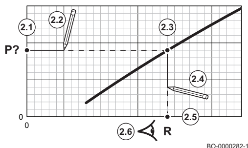
Εικ.66 Ισχύς που απαιτείται
