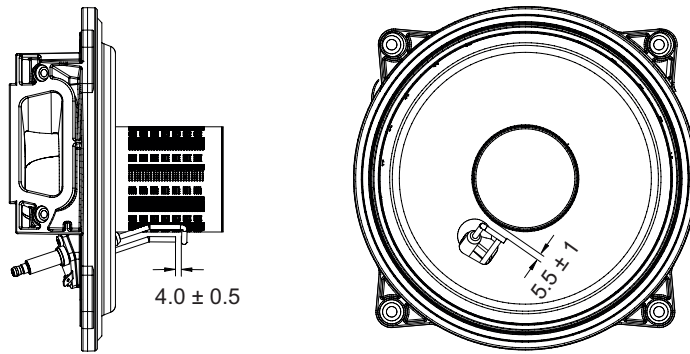
Εικ.74 Απόσταση ηλεκτροδίου
