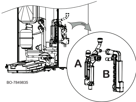
Εικ.73 Αποσυναρμολόγηση του σιφονιού
