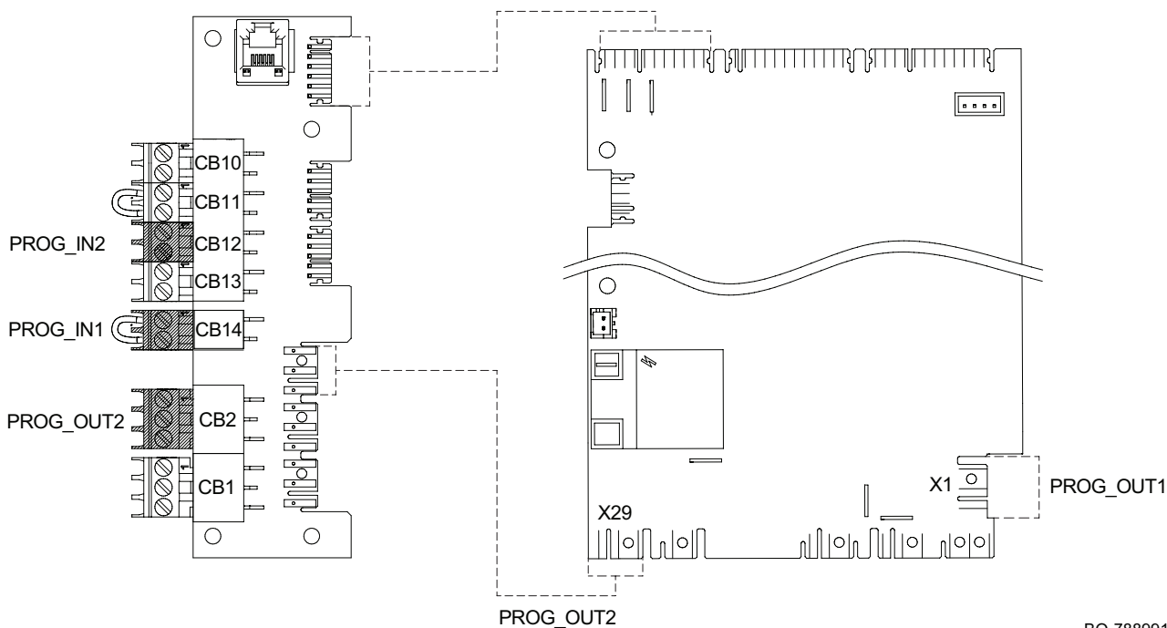
Εικ.50 Διάταξη παραμετροποίησης προγραμματιζόμενων εισόδων και εξόδων
