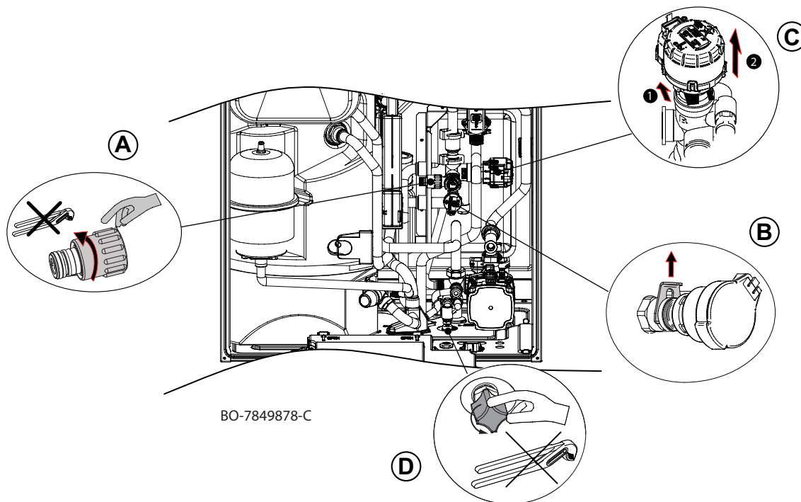
Εικ.75 Βασικά εξαρτήματα υδραυλικής μονάδας
