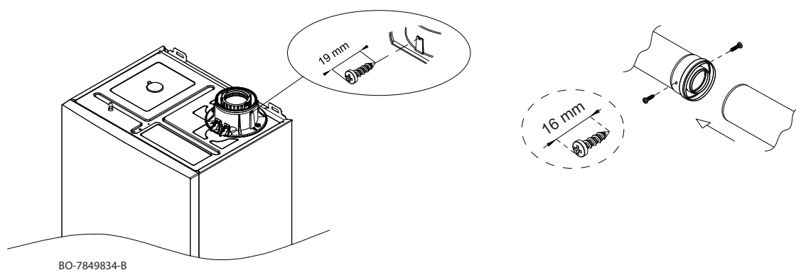
Εικ.40 Ομοαξονική στερέωση πύργου καπναερίων
