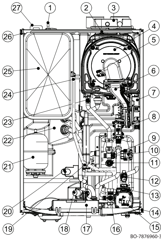
Εικ.26 Περιγραφή εξαρτημάτων
