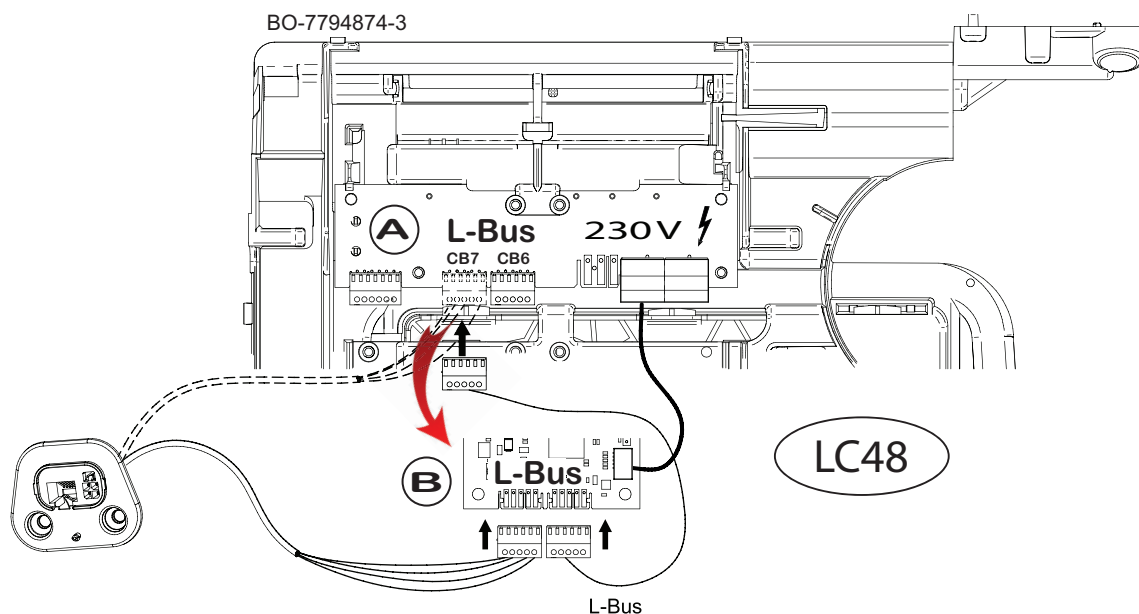
Εικ.49 Σύνδεση της πλακέτας παρελκομένων στον λέβητα
