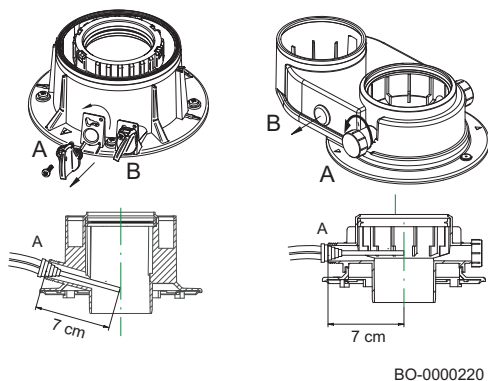
Εικ.59 Τύπος συνδέσεων — σημείο μέτρησης καπναερίων
