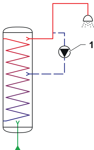
Εικ.51 Σύνδεση κυκλοφορίας ZNOX
