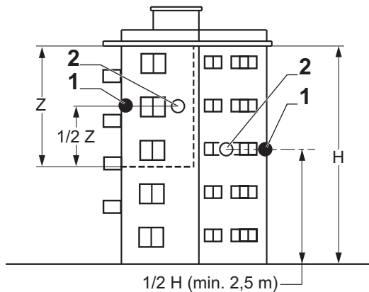
Εικ.33 Συνιστώμενα σημεία Α
