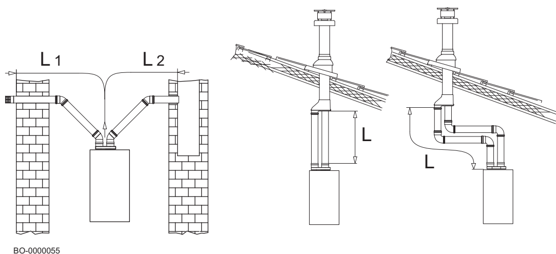
Εικ.44 Παραδείγματα εγκατάστασης ξεχωριστών σωλήνων
