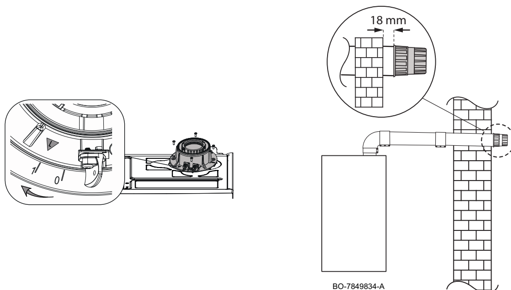
Εικ.38 Εγκατάσταση ομόκεντρου εξαρτήματος
