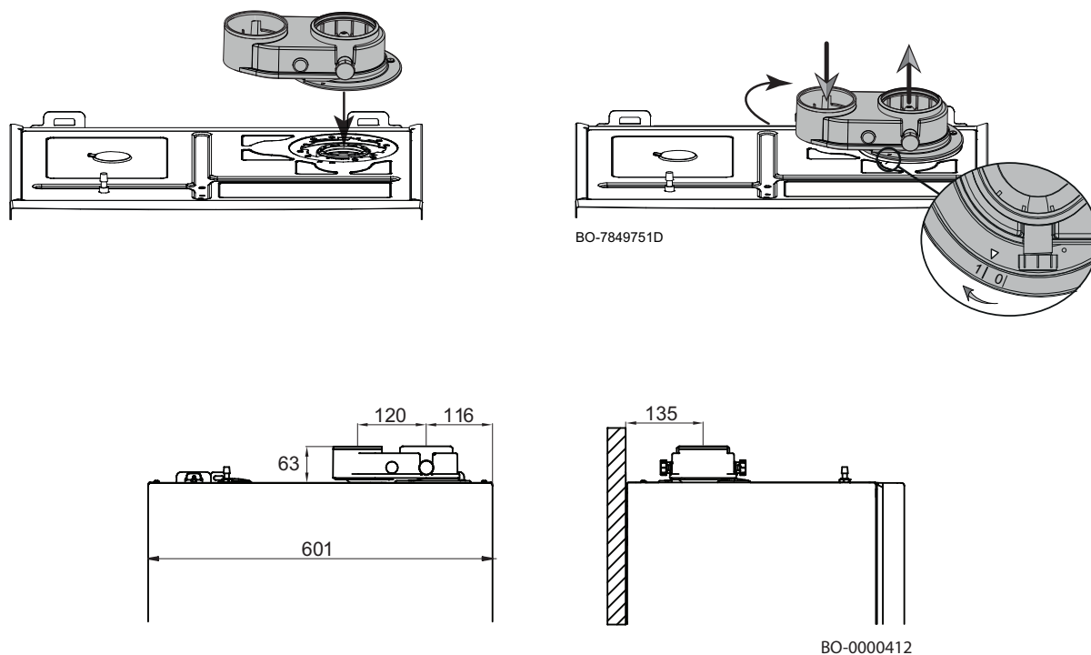
Εικ.43 Εγκατάσταση ξεχωριστών σωλήνων
