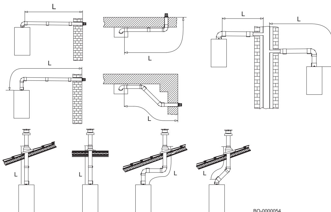
Εικ.41 Παραδείγματα εγκατάστασης ομόκεντρων σωλήνων
