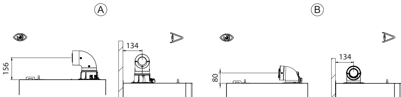
Εικ.39 Εισαγωγή-εξαγωγή ομόκεντρου τύπου
