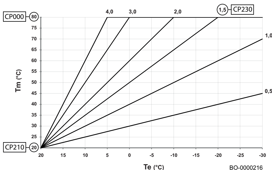
Εικ.70 Γραφική παράσταση καμπύλης θέρμανσης
