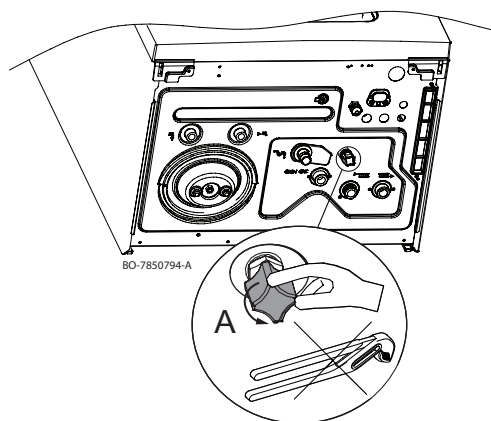
Εικ.20 Πλήρωση της εγκατάστασης
