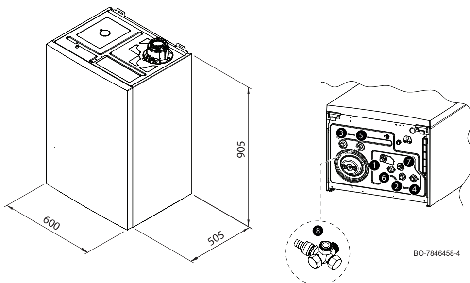
Εικ.22 Διαστάσεις και συνδέσεις
