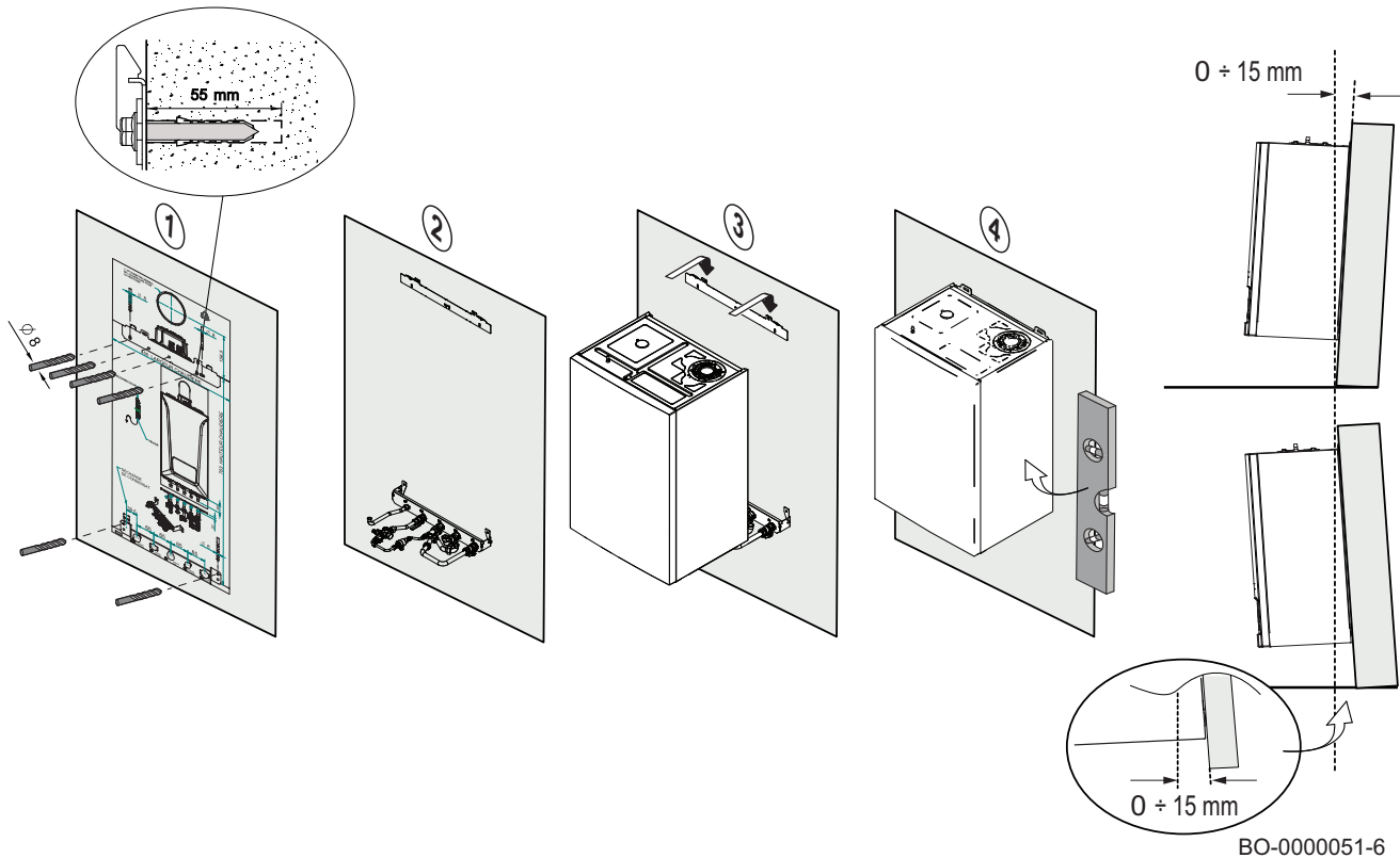
Εικ.32 Επιτοίχια εγκατάσταση του παρελκομένου
