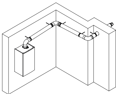
Εικ.36 Μέθοδος στερέωσης των σωλήνων στον τοίχο
