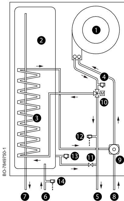
Εικ.25 Σχηματικό διάγραμμα
