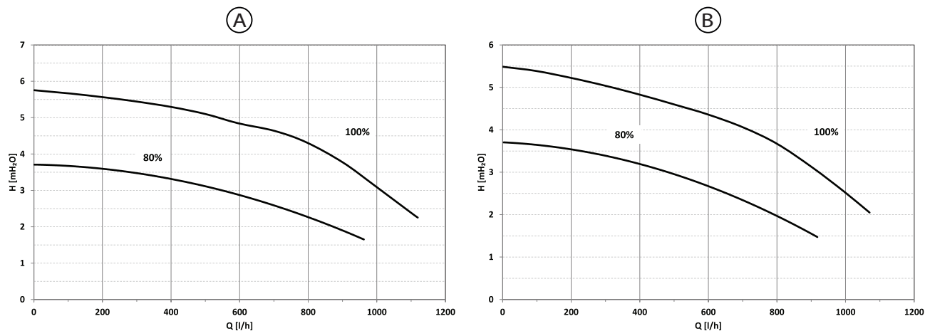
Εικ.27 Γράφημα παροχής/μανομετρικού ύψους στην πινακίδα
