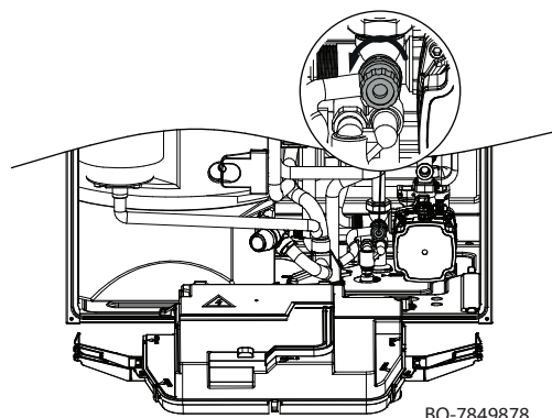
Εικ.56 Εκκένωση της εγκατάστασης
